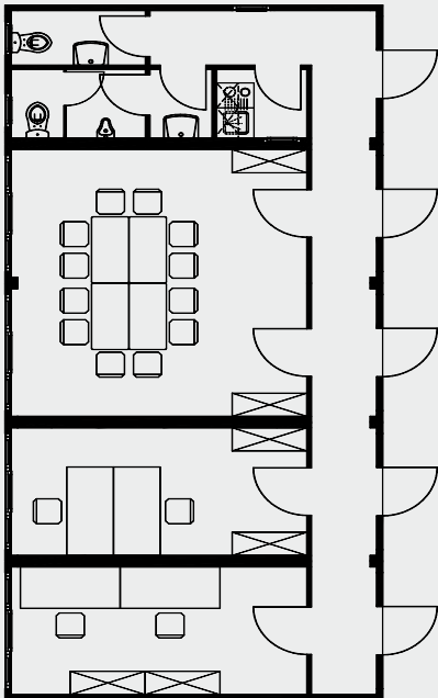
Grundrissbeispiel: Baustellenbüro
